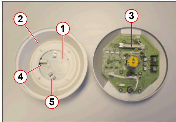
Fig. 356: Alarm box
