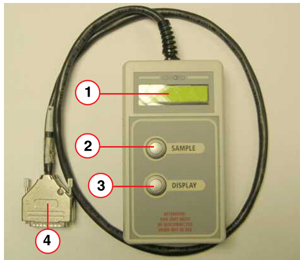
Fig. 375: MSUP- Display Unit
